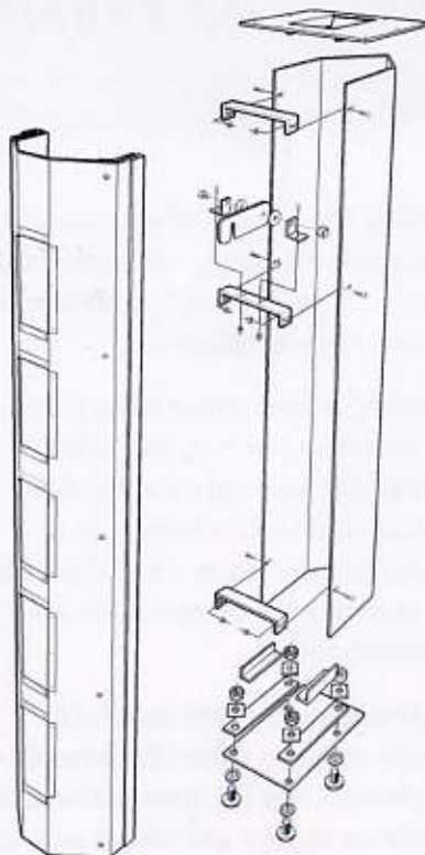
Ducto central para la entrada del aire
